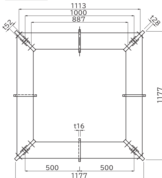
寸法図
