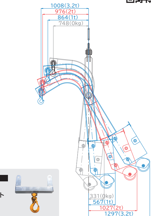
荷重曲線図
