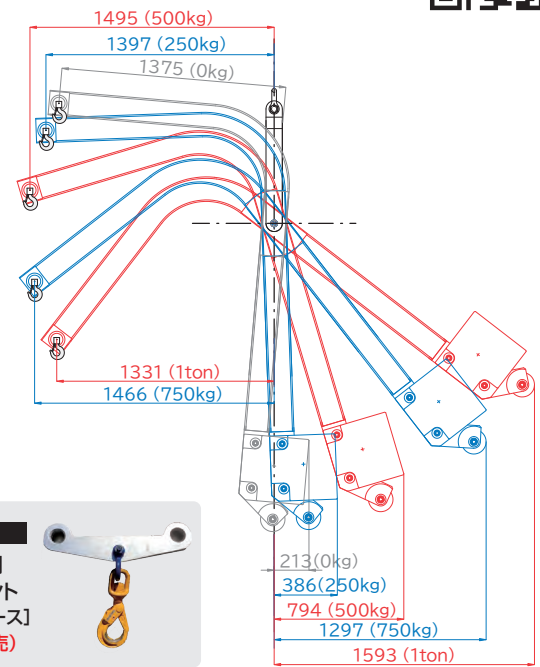
荷重曲線図
